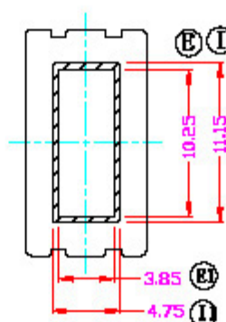
A-A SECTION
